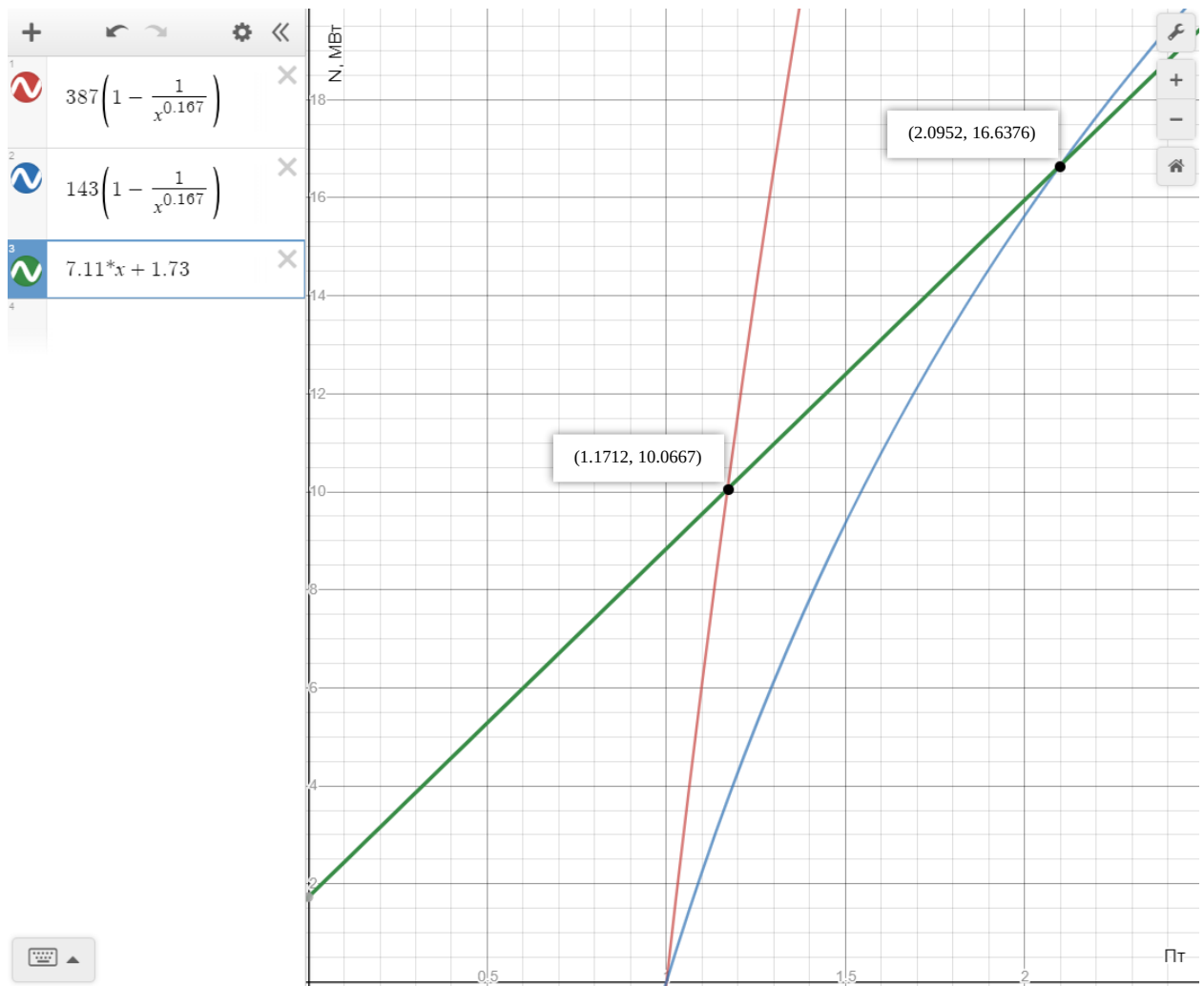
Рис.1. Зависимость N(\pi_T) , где N_H(\pi_T) обозначен зеленым цветом, N_{OГГ}(\pi_T) - красным цветом, N_{BГГ}(\pi_T) - синим цветом.
